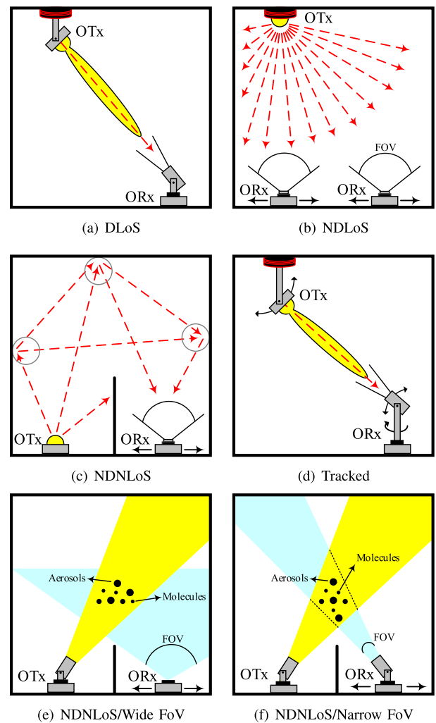
Fig. 2. OWC channel scenarios.
